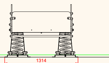
PERFIL
