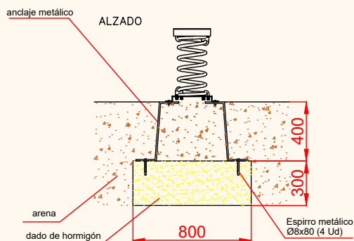
DETALLES DE CIMENTACIÓN ESQUEMA DE CIMENTACIÓN EN ARENA
