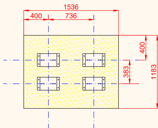
PLANO DE CIMENTACIÓN
