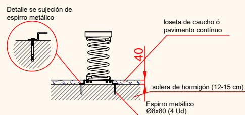
ESQUEMA DE CIMENTACIÓN EN HORMIGÓN
