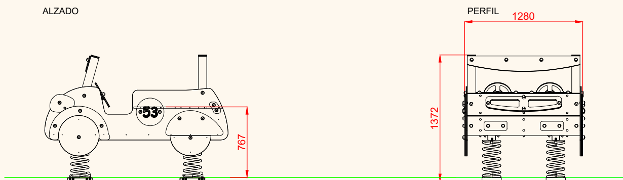
ALZADO
