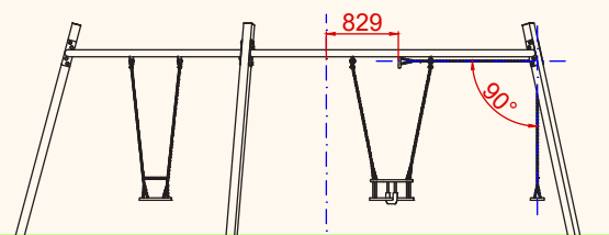
PERFIL
