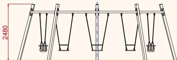
ALZADO
