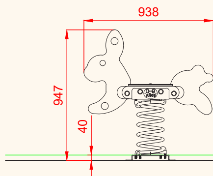
ALZADO
