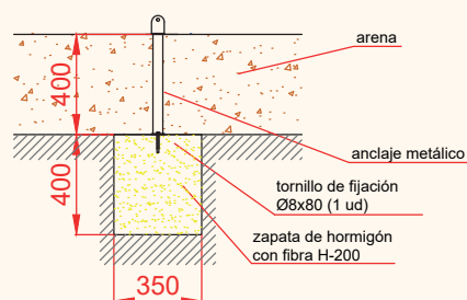
ESQUEMA DE CIMENTACIÓN EN ARENA
