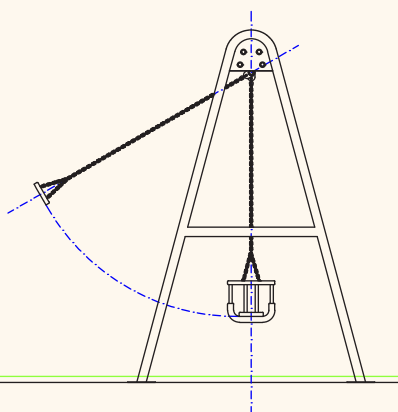
PERFIL
