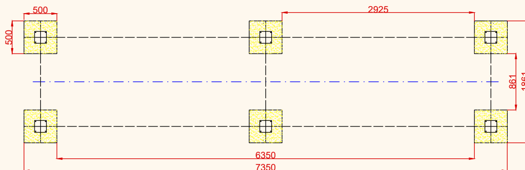
DETALLES CIMENTACIÓN
