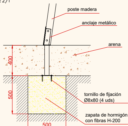
DETALLES CIMENTACIÓN
