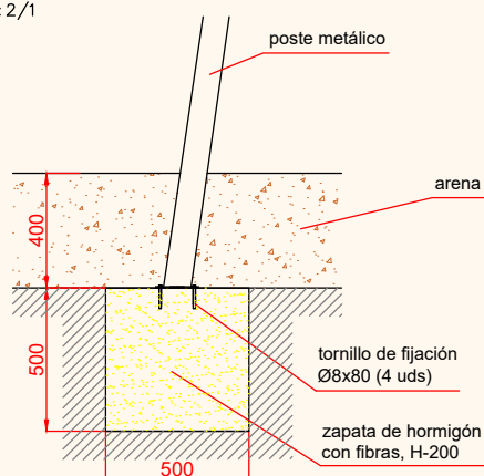
ESQUEMA DE CIMENTACIÓN EN ARENA E: 2/1
