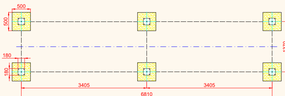
DETALLES CIMENTACIÓN
