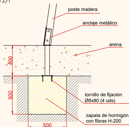
DETALLES CIMENTACIÓN
