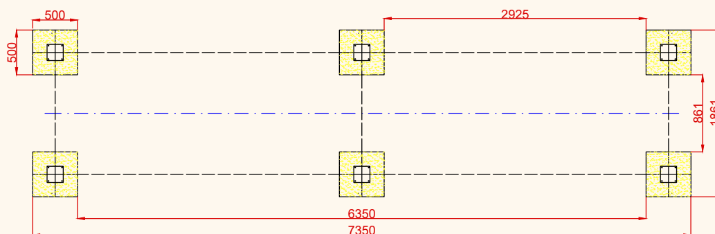
DETALLES CIMENTACIÓN
