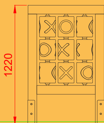
ALZADO
