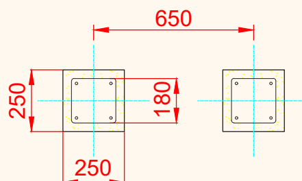
PLANTA CIMENTACIÓN
