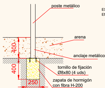
DETALLES CIMENTACIÓN
