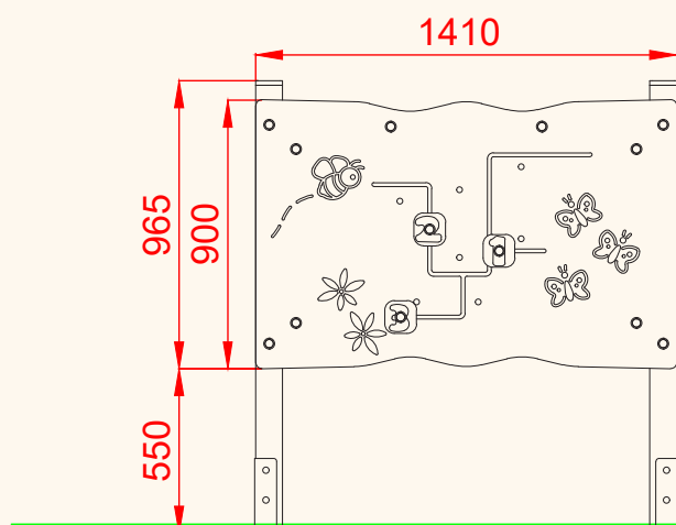
ALZADO
