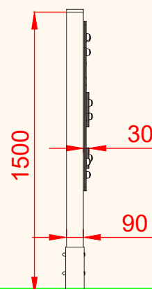
PERFIL IZQUIERDO
