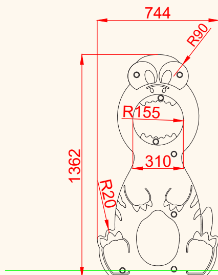
ALZADO
