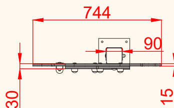
PLANTA
