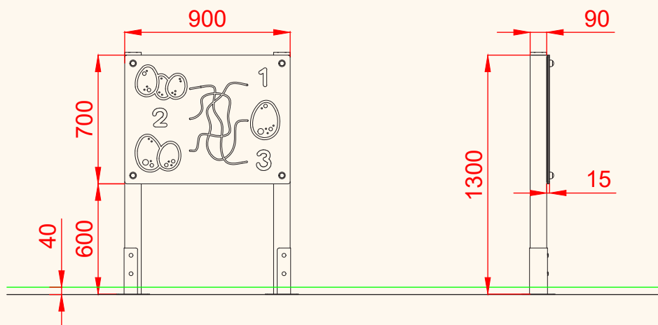
ALZADO
