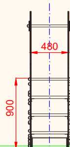
PERFIL IZQUIERDO
