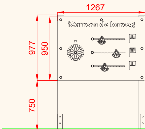
ALZADO
