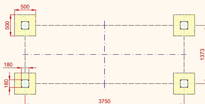
PLANTA CIMENTACIÓN
