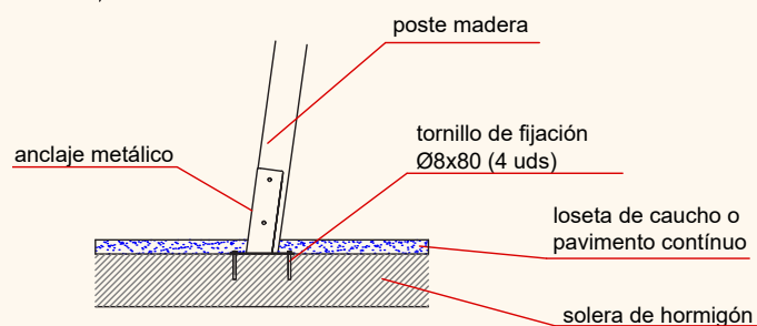
ESQUEMA DE CIMENTACIÓN EN HORMIGÓN
