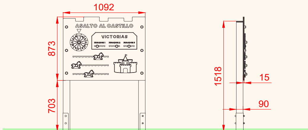
PERFIL IZQUIERDO
