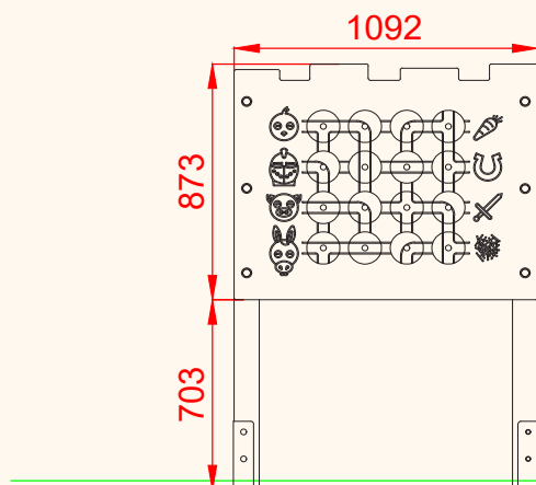
ALZADO
