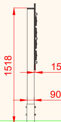
PERFIL IZQUIERDO
