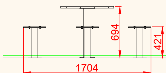
ALZADO
