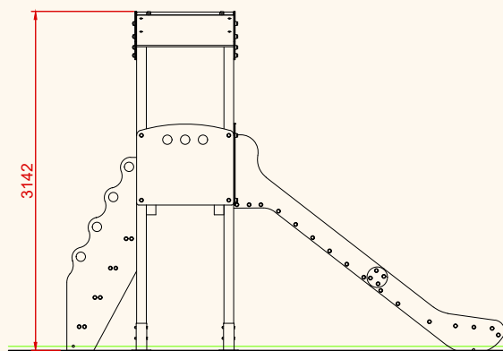
ALZADO
