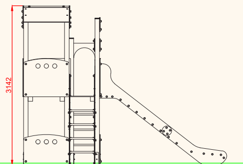
PERFIL
