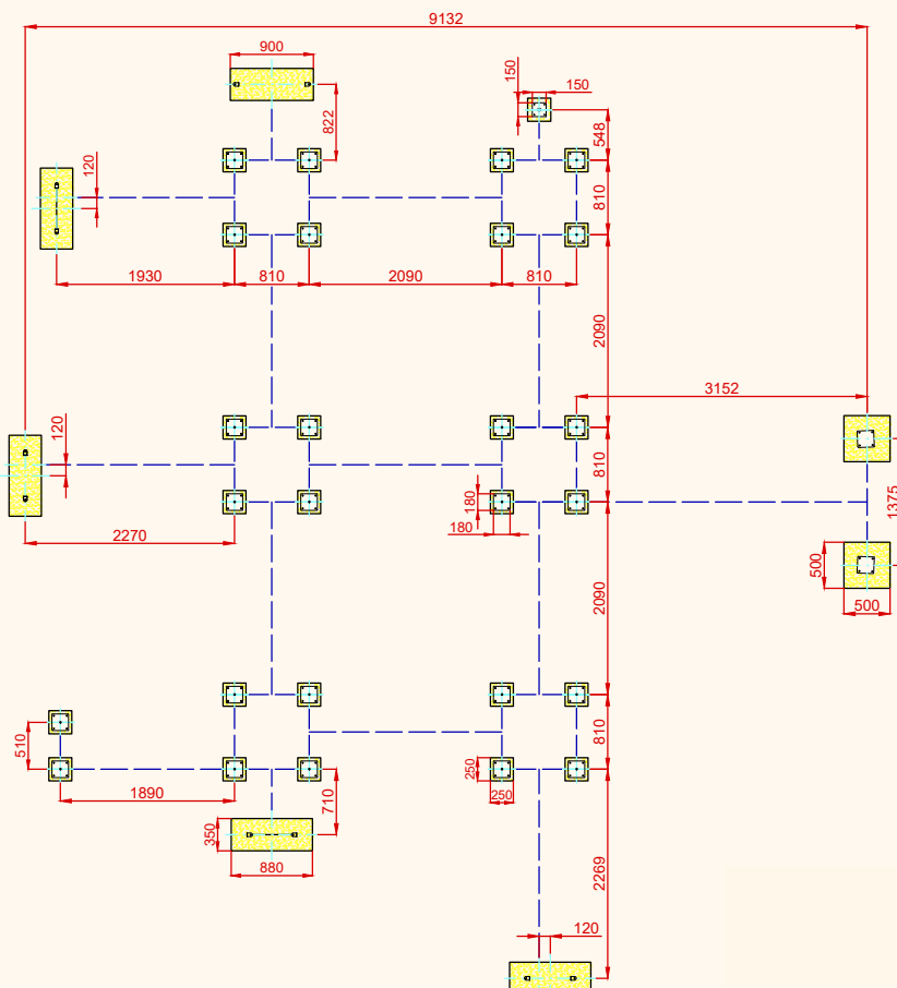
PLANTA CIMENTACIÓN
