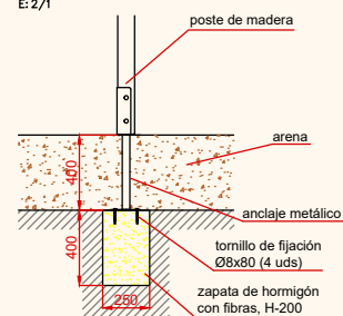
DETALLES CIMENTACIÓN
