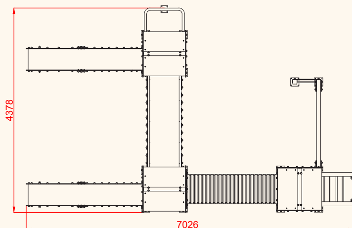
PLANTA
