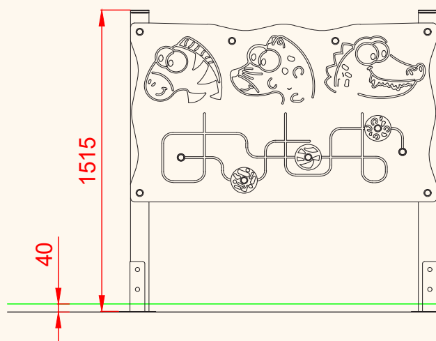
ALZADO
