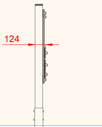
PERFIL IZQUIERDO
