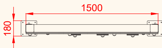
PLANTA
