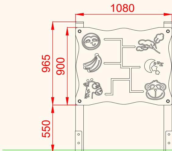
ALZADO
