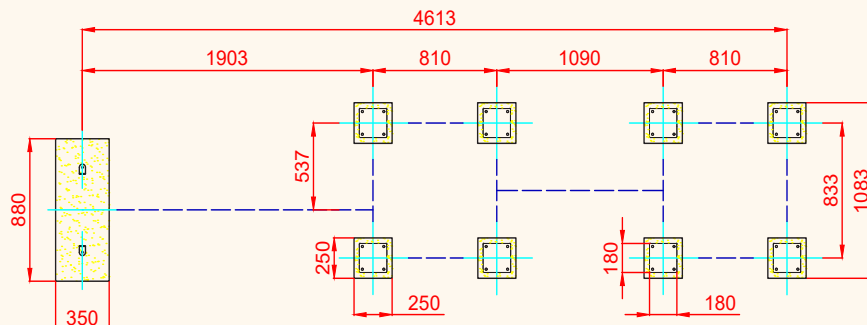
PLANTA CIMENTACIÓN
