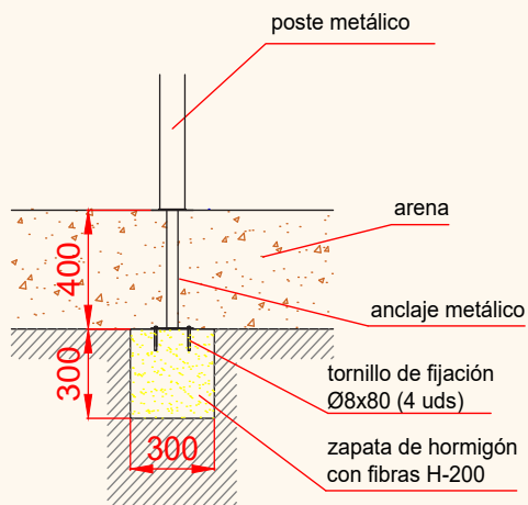
DETALLES CIMENTACIÓN ESQUEMA DE CIMENTACIÓN EN ARENA
