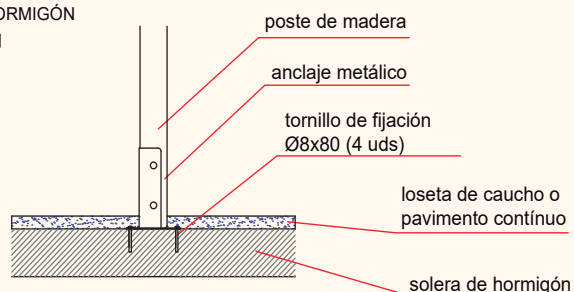
ESQUEMA DE CIMENTACIÓN EN HORMIGÓN
