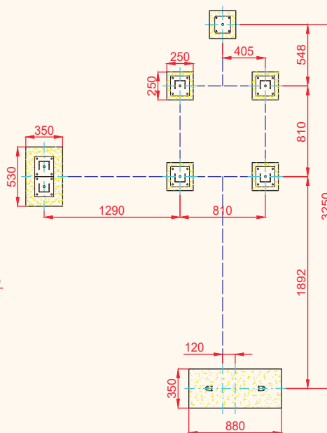
PLANTA CIMENTACIÓN
