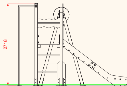
PERFIL IZQUIERDO
