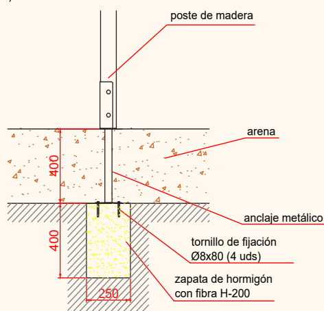
ESQUEMA DE CIMENTACIÓN EN HORMIGÓN
