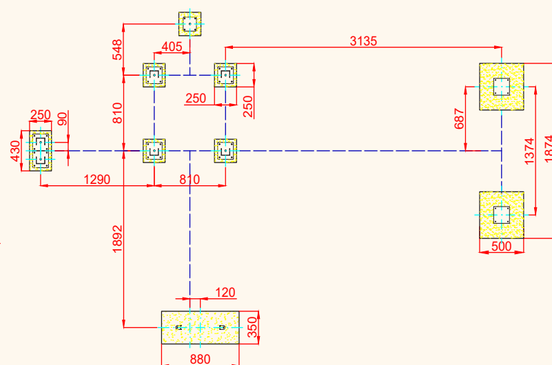
PLANTA CIMENTACIÓN
