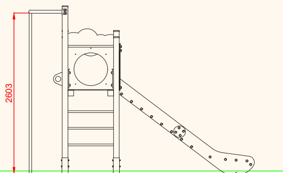
PERFIL IZQUIERDO
