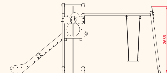
ALZADO
