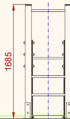
PERFIL IZQUIERDO
