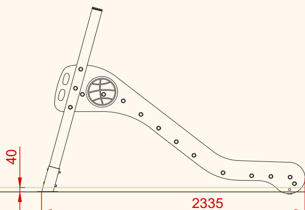
ALZADO
