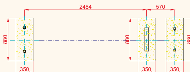
PLANTA CIMENTACIÓN
