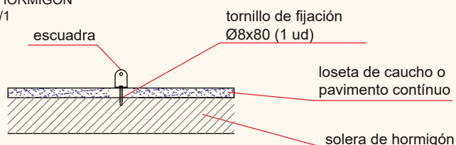
ESQUEMA DE CIMENTACIÓN EN HORMIGÓN E: 2/1
