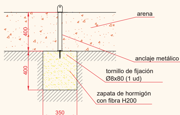
ESQUEMA DE CIMENTACIÓN EN HORMIGÓN E: 2/1
