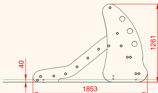
ALZADO
