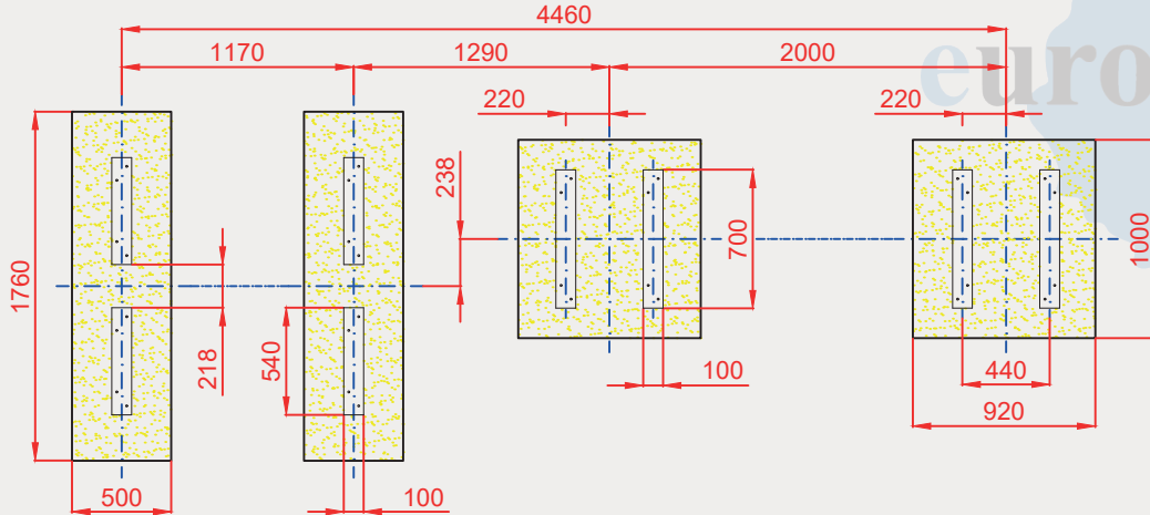
PLANTA CIMENTACIÓN
