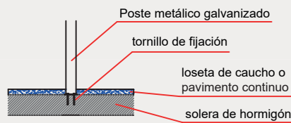
ESQUEMA DE CIMENTACIÓN EN HORMIGÓN
