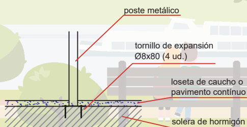
DETALLE DE ANCLAJE
