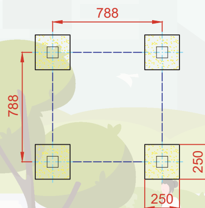
PLANTA CIMENTACIÓN
